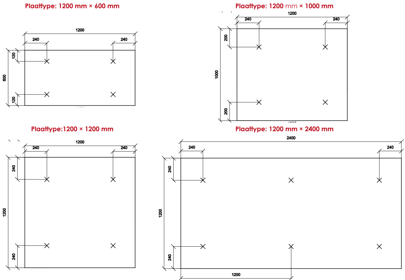
Fig. 1 plaatsingspatroon voor de mechanische bevestigingen
